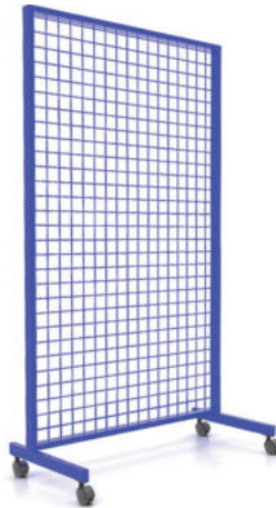
ขนาด 90 x 150 ซม. ลวด 3 มม.
